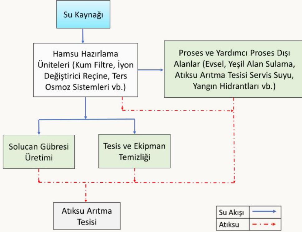
Diğer Hayvan Yetiştiriciliği Sektörü Su Akım Şeması
