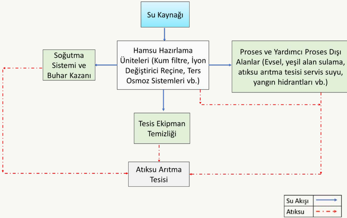
Birincil Formda Sentetik Kauçuk İmalatı Sektörü Su Akım Şeması
