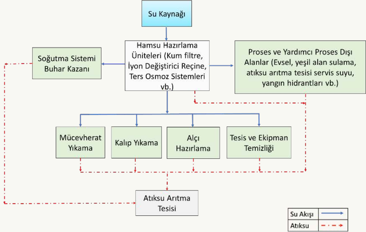
Mücevher ve Benzeri Eşyaların İmalatı Sektörü Su Akım Şeması
