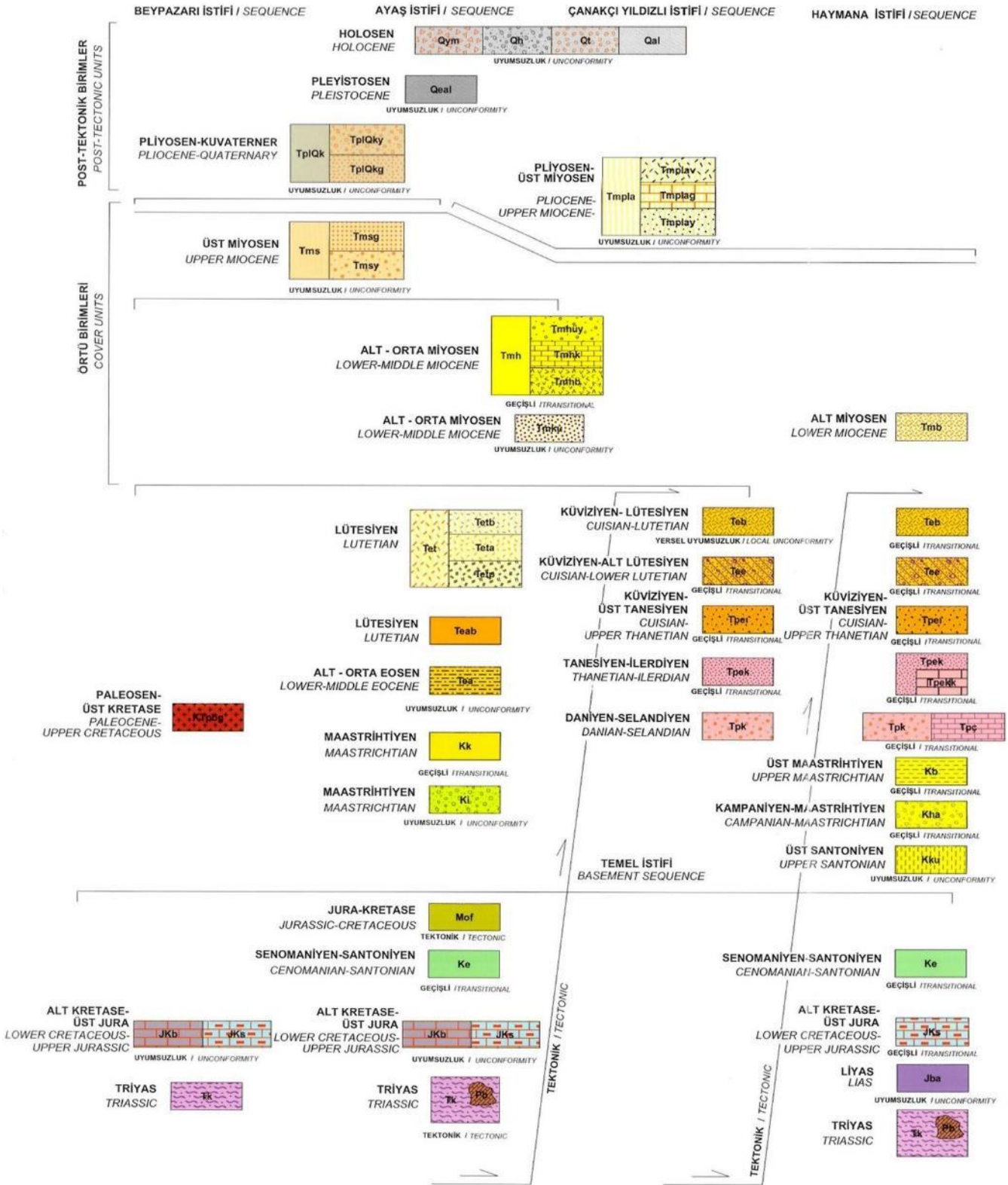
Şekil 28 Proje Alanı ve Çevresinin Genelleştirilmiş Stratigrafik Sütun Kesiti
