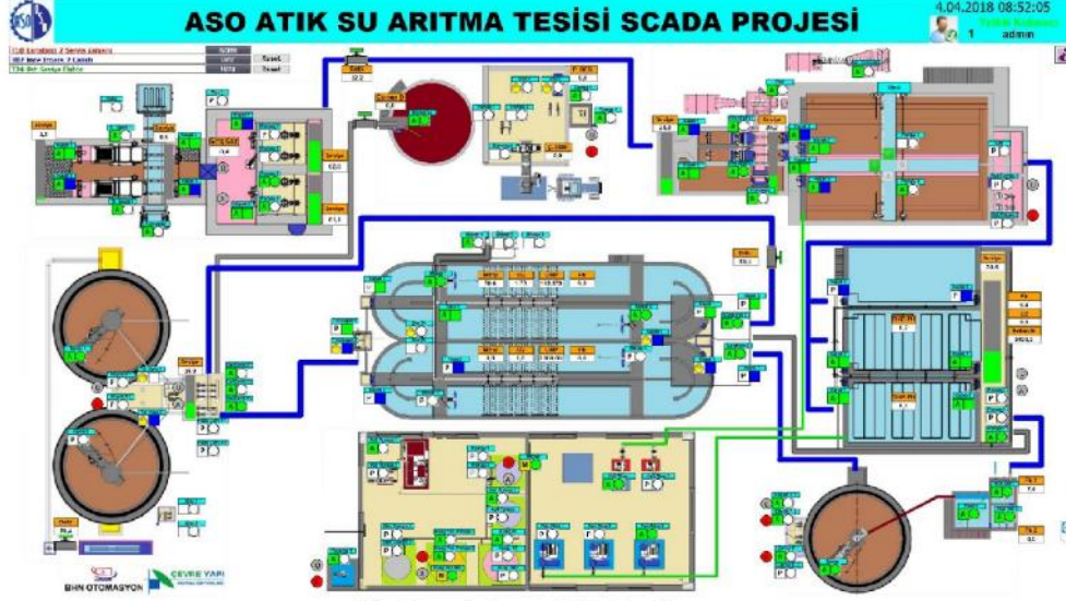
3.1. Atıksu Arıtma Tesisi İş Akım Şeması
