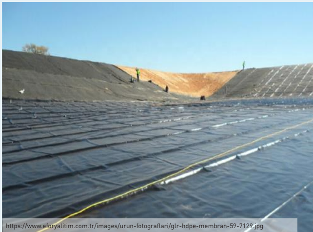
Maden Atık Barajı İnşaatı Geomembran Uygulaması
