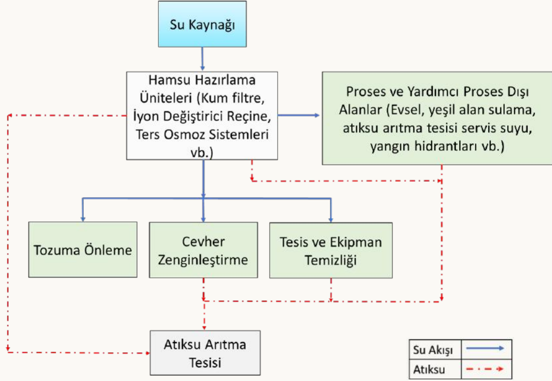
Demir Cevherleri Madenciliği Sektörü Su Akım Şeması
