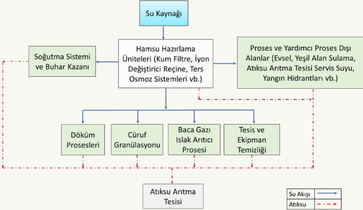
Diğer Demir Dışı Metallerin Dökümü Sektörü Su Akım Şeması
