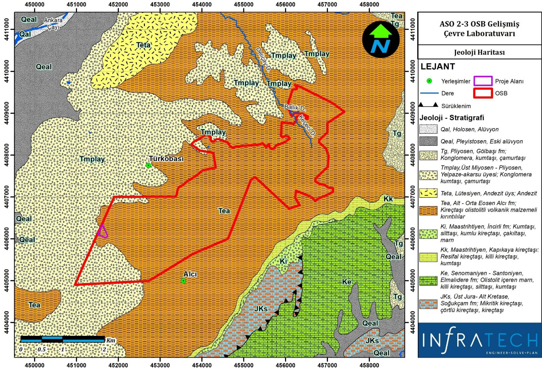
Şekil 29 Proje Alanının Jeoloji Haritası
